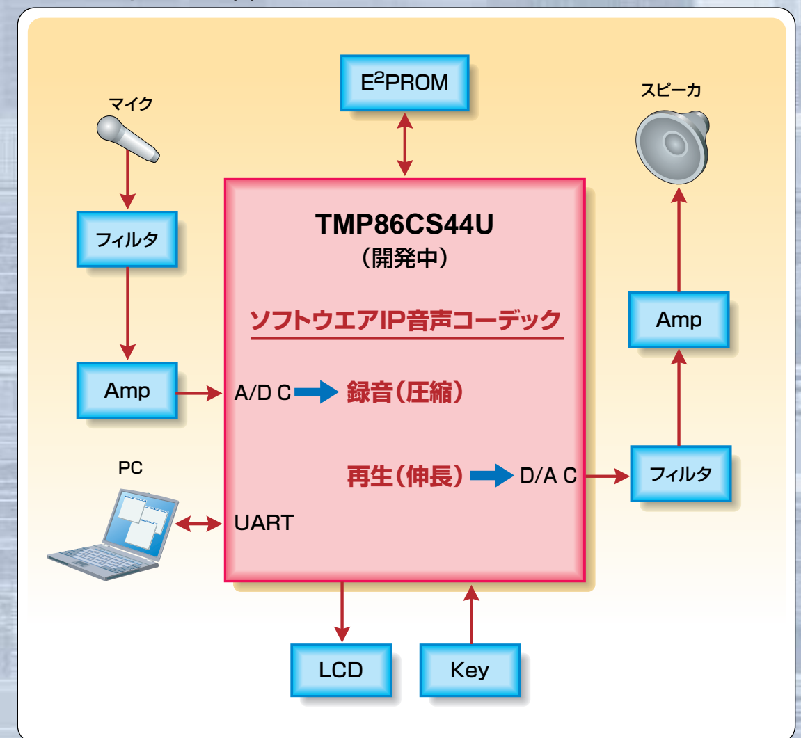
■ デモボード ブロック図
