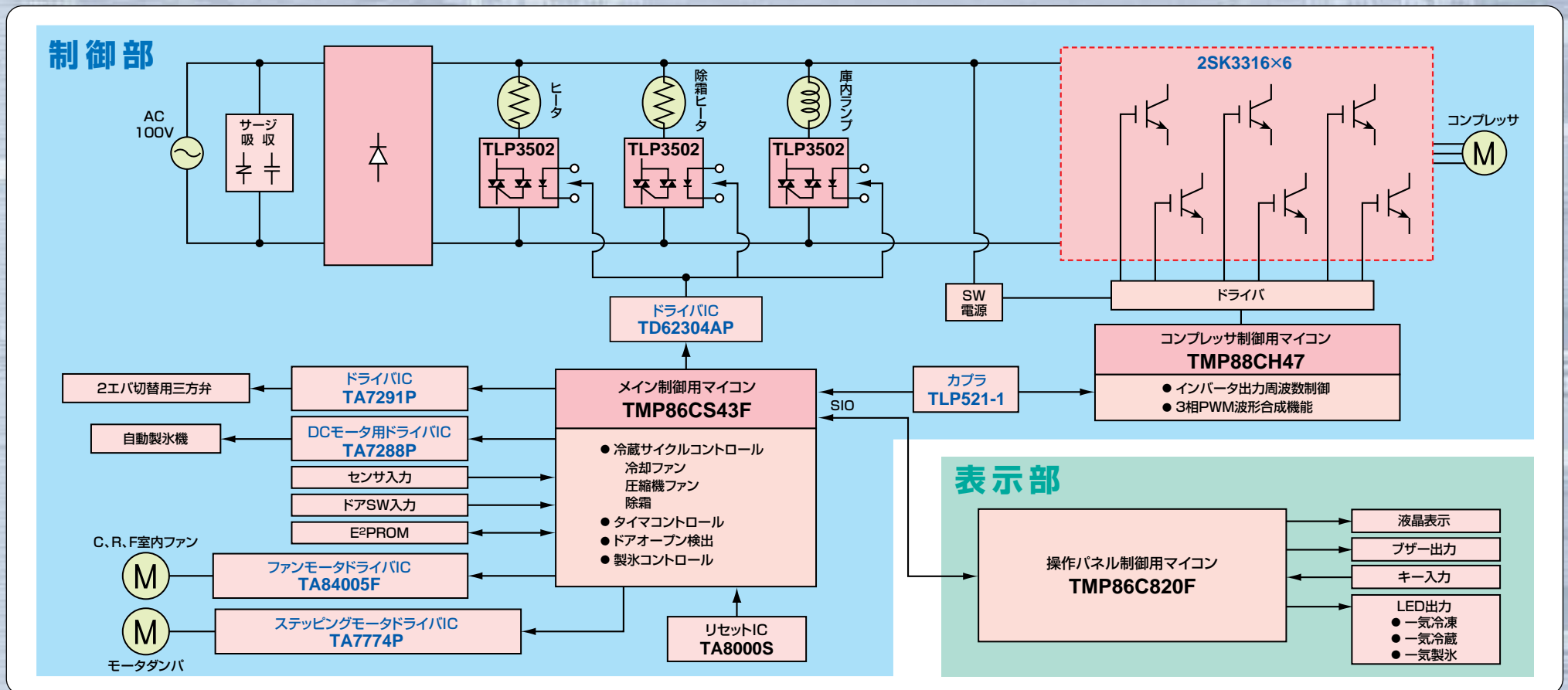
■ インバータ冷蔵庫ブロック図
