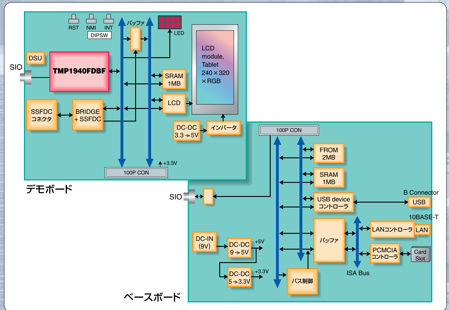
■TMP1940リファレンスボード
