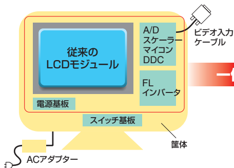
従来のLCDモジュールを採用したセット
